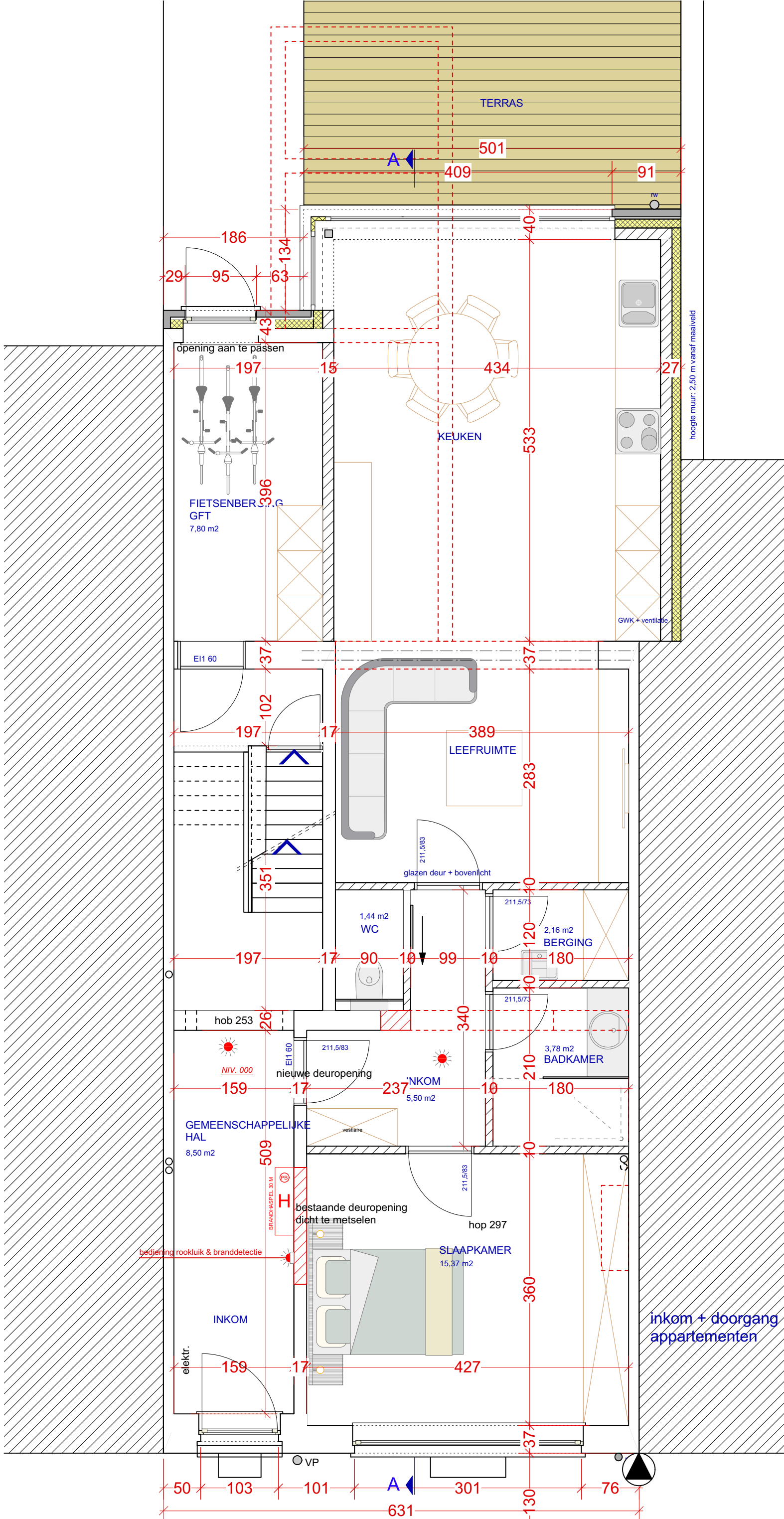
GRONDPLAN NIEUWE TOESTAND voetpad - klinkers
